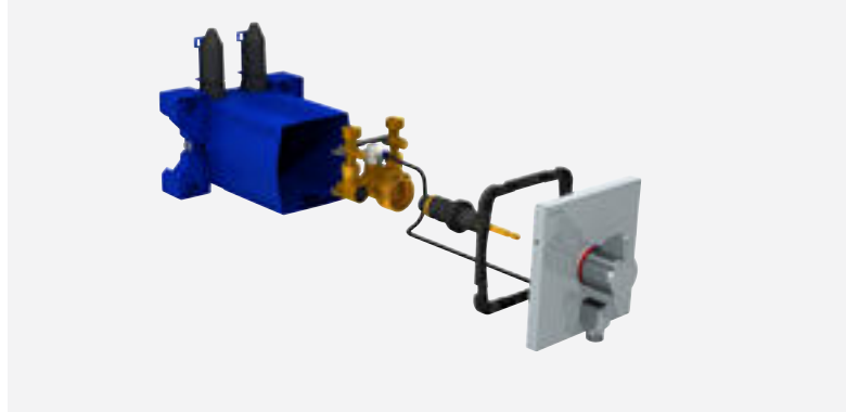
Brause-Thermostatarmatur für Unterputzmontage Art. DELABIE: H96CBOX + H9633
